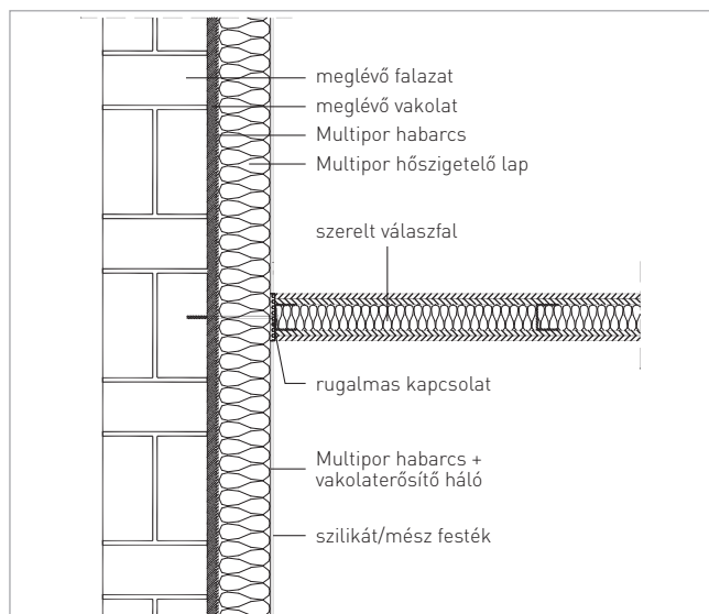
Szerelt válaszfal – vízszintes (b)
