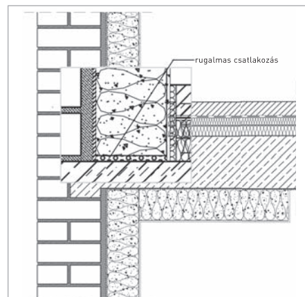
Rugalmas csatlakozás – padló
