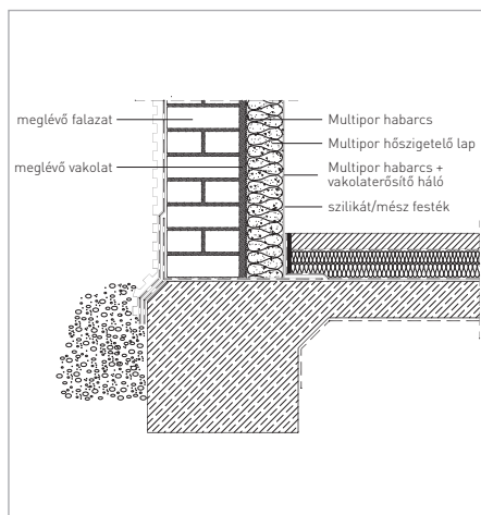
Padlócsatlakozás
