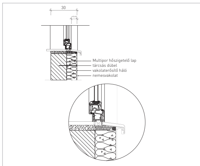
Nyílászáró – függőleges
