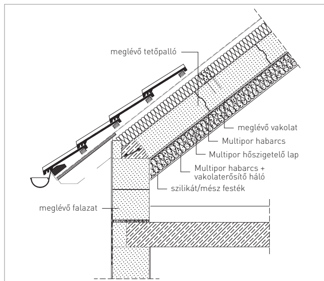
Tetőtér pallófödém 3.
