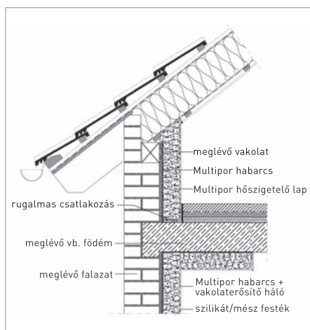
Tetőtér beépítés
