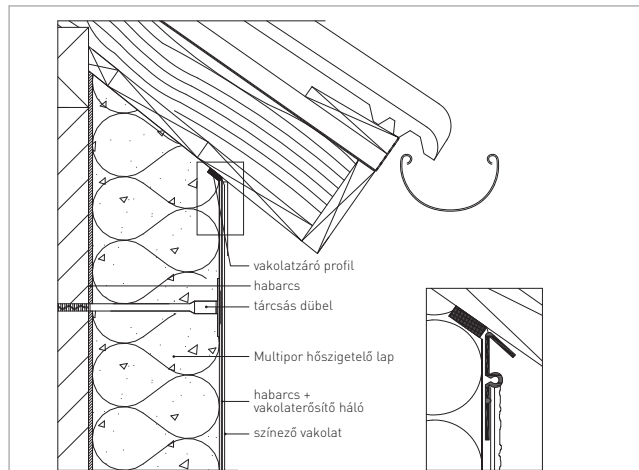
Ereszcsatlakozás 2.
