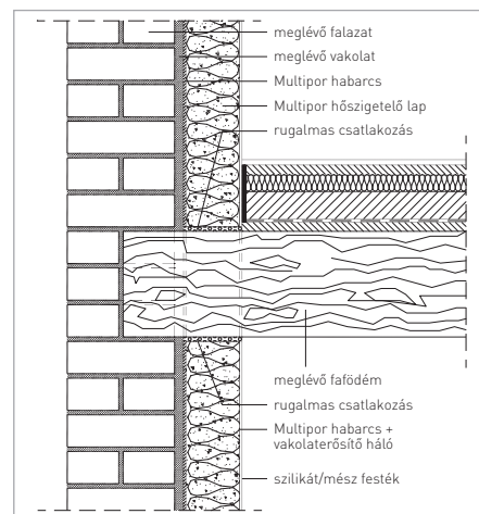
Födémcsatlakozás 2.
