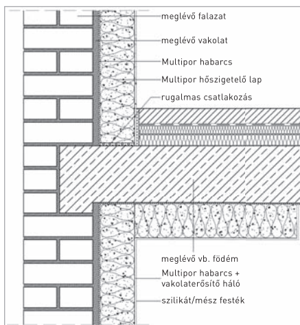
Födémcsatlakozás 1.
