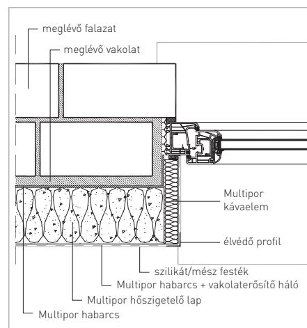
Ablakkáva, vízszintes
