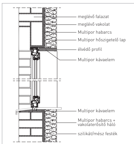
Ablakkáva, függőleges
