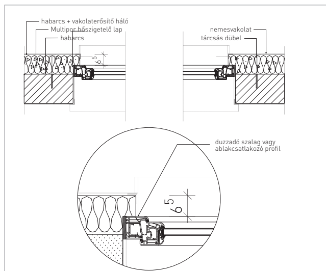
Nyílászáró – vízszintes
