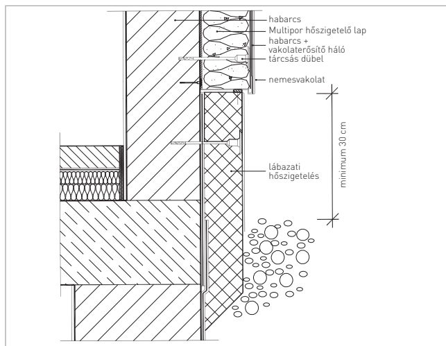
Lábazatkialakítás
