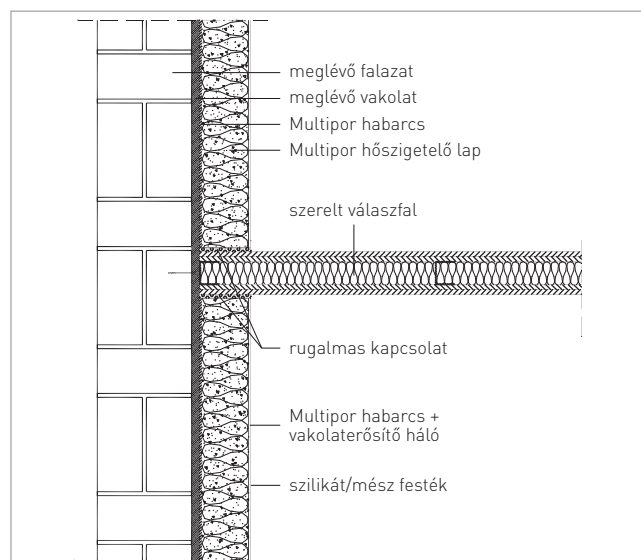
Rétegrend
