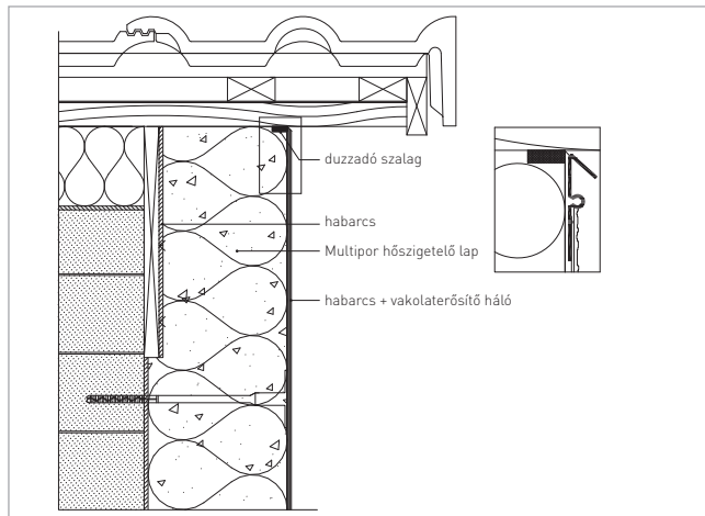
Ereszcsatlakozás 1.
