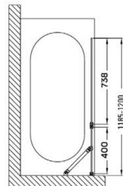
EDGE 120 KÁDPARAVÁN
