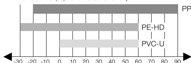
Hőmérséklet (°C) – alkalmazási tartomány
