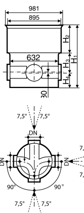
Tegra 800 aknafenek – elágazó 90°
