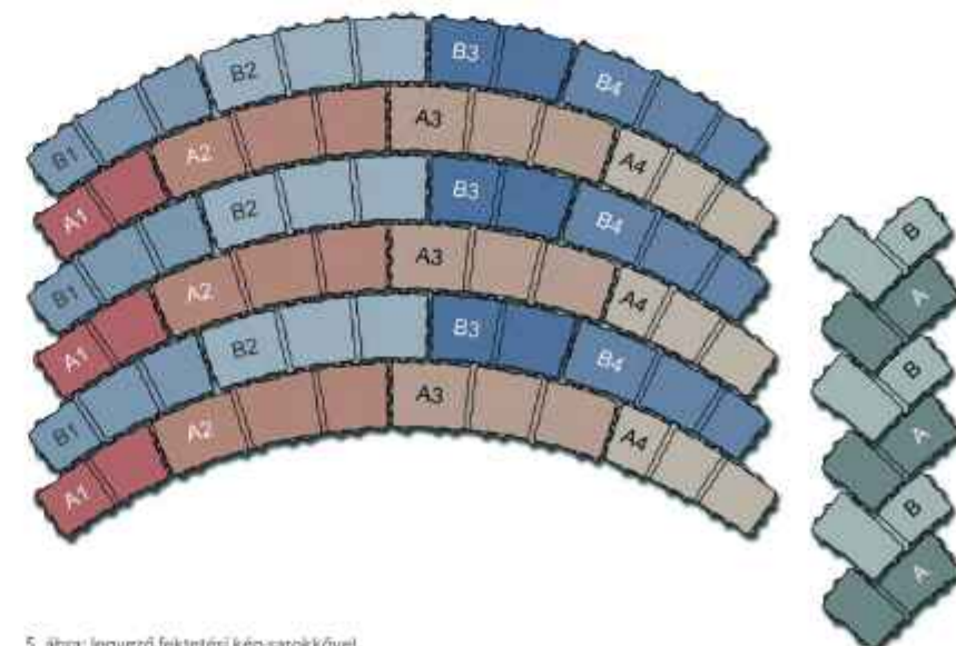
5. ábra: legyenek fedtetési kép-sarokkövel
