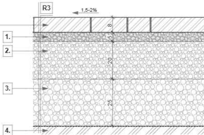
Térkö burkolat 8 cm vtg. teher forgalom számára
