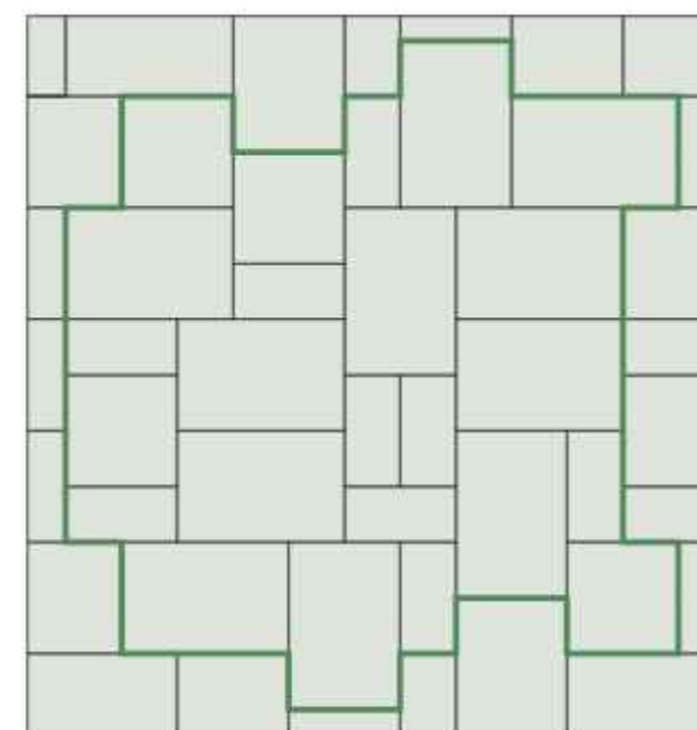
10. minta Méret 20×40 cm 40×40 cm 40×60 cm Igény/m 2 kb. 2,25 db kb. 1 db kb. 2,75 db
