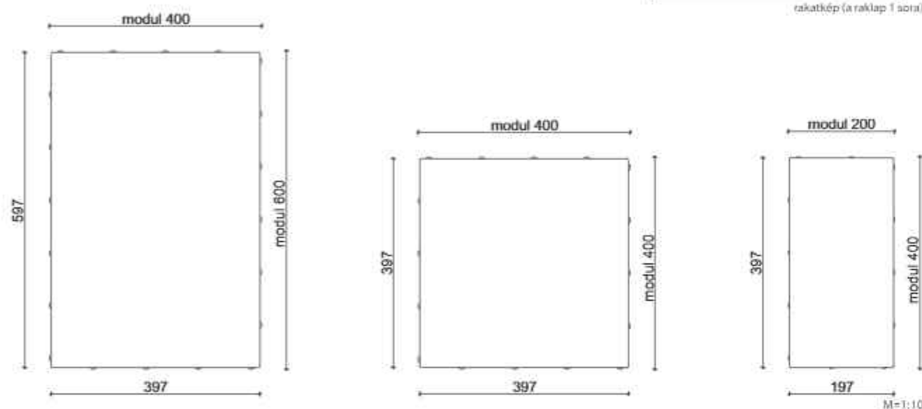
rakatkép (a raklap 1 sora)
