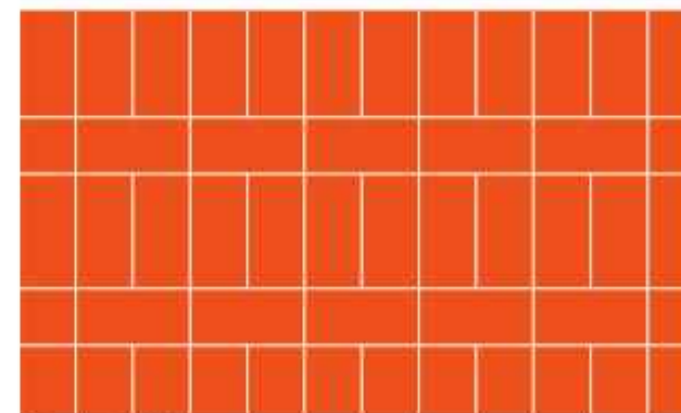
Futósoros és vállkötés
