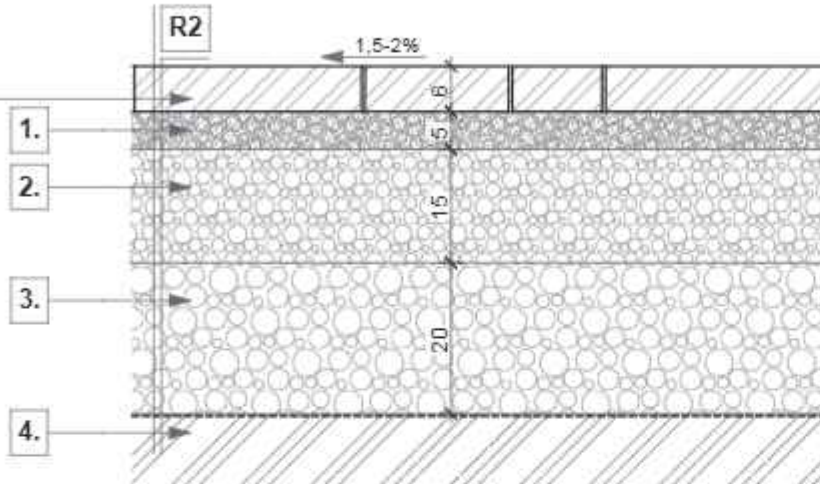
Térkö burkolat 6 cm vtg. gépjármű forgalom számára
