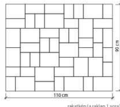
rakatkép (a raklap 1 sora)
