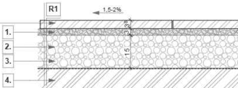
Lap burkolat gyalogos forgalom számára
