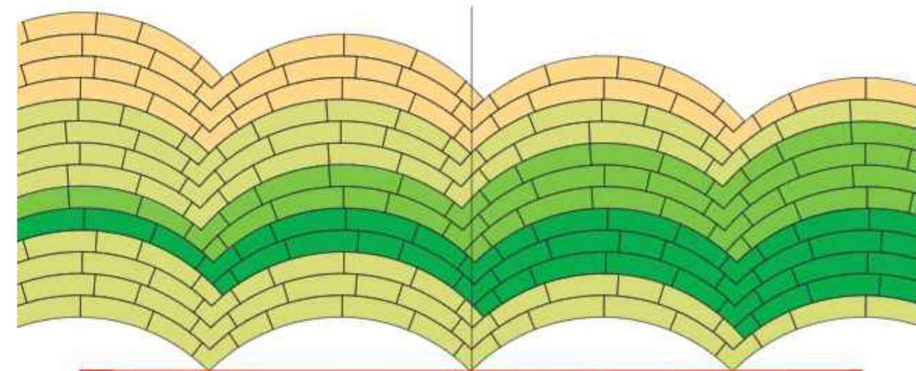
21. ábra: 1 jobbos - 2 balos - 2 jobbos lerakási egység kialakítása
