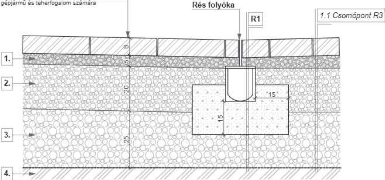
Semmelrock térkő burkolat 8 cm vtg. gépjármű és teherfoglalom számára
