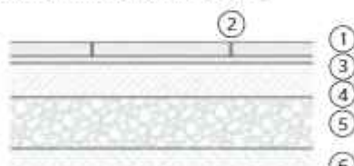
Lapok fektetése habarcságyra (gyalogos forgalmú felületek)
