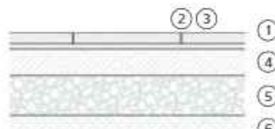
Lapok fektetése laptartó tappancsra (csak gyalogos forgalmú felületek)
