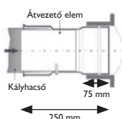
Füstcső-csatlakozó T-idomhoz, tömítő szalaggal
