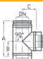
T-idom 90 fokos
