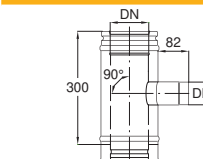
T-idom 90 fokos 80 mm-es csatlakozással
