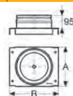
Közbső támasz
