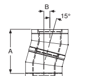
Könyök 15°
