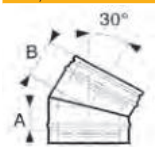
Könyök 30 fokos
