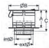
Esővédő gallér
