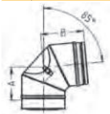
Könyök 85 fokos vizsgálónylással
