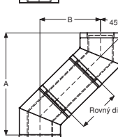
Könyök 45° csőelemmel
