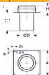
Talpelem kéménytoldáshoz UNI-ICS50
