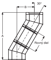
Könyök 30° csőelemmel
