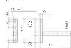
Falkonzol hosszú (pár)
