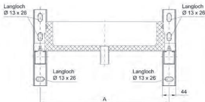
Méretek a 325-től a 475-ös típusok esetén
