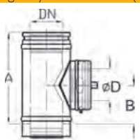
Vizsgálónyílásos elem P1 (rövid)
