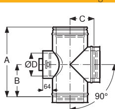
T-idom 90 fokos N1 vizsgáló nyílással
