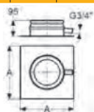
Talplemez konzolos szereléshez
