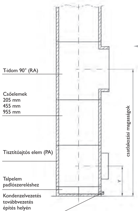
Csatlakozási magasságok padlóról való indítás esetén
