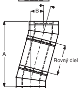
Könyök 15° csőelemmel
