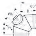
Könyök 85 fokos P1 vizsgálónylással
