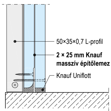
W628-A Aljzatcsatlakozás
