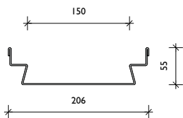
BG-PA SV NM 150 gyorscsatlakozó rendszerrel
