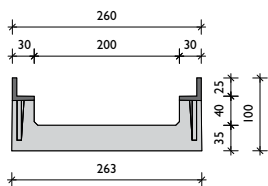
BGF-Z SV 200 öntöttvas tokkal
