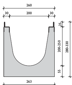
BGU-Z SV 200 rozsdamentes vagy horganyzott acél tokkal
