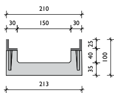
BGF-Z SV 150 öntöttvas tokkal
