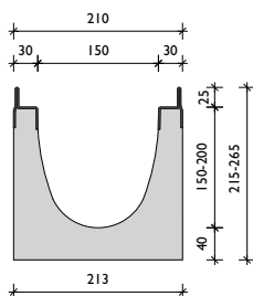
BGU-Z SV 150 rozsdamentes vagy horganyzott acél tokkal
