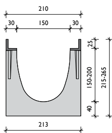
BGU-Z SV 150 öntöttvas tokkal
