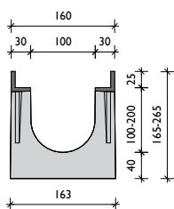
BGU-Z SV 100 öntöttvas tokkal
