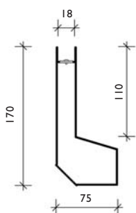
BG-FA Homlokzati résfolyóka RSZ 18
