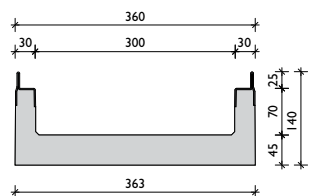
BGF-Z SV 300 rozsdamentes vagy horganyzott acél tokkal
