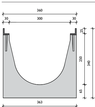
BGU-Z SV 300 öntöttvas tokkal
