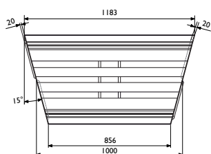
Flex kábelcsatorna méret 3
