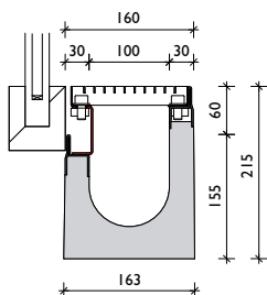
BGU-Z Homlokzati folyóka
