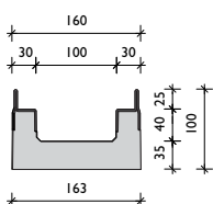
BGF-Z SV 100 rozsdamentes vagy horganyzott acél tokkal
