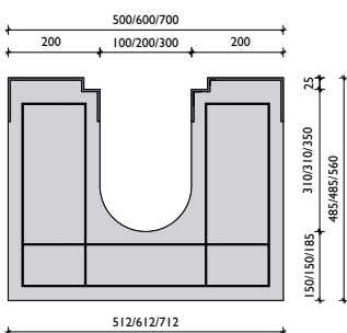
BG-SI Biztonsági folyóka névleges méret 100, 200 vagy 300
