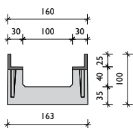
BGF-Z SV 100 öntöttvas tokkal
