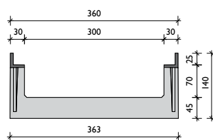
BGF-Z SV 300 öntöttvas tokkal
