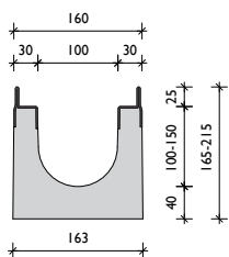
BGU-Z SV 100 rozsdamentes vagy horganyzott acél tokkal
