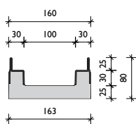
BGF-Z SV 100 rozsdamentes vagy horganyzott acél tokkal
