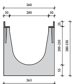
BGU-Z SV 200 öntöttvas tokkal
