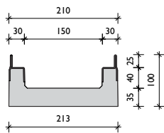
BGF-Z SV 150 rozsdamentes vagy horganyzott acél tokkal
