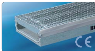
BGF-Z SV 300 öntöttvas tokkal
