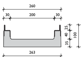
BGF-Z SV 200 rozsdamentes vagy horganyzott acél tokkal
