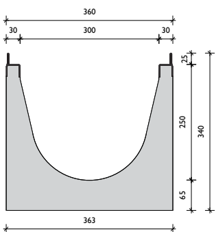
BGU-Z SV 300 rozsdamentes vagy horganyzott acél tokkal
