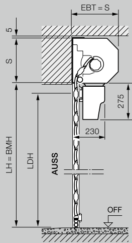
Belső és külső szerelésű redőnykapuk mérettartománya
