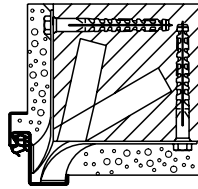
Saroktok Beépítés téglafalba Horgony
