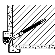
Speciális saroktok Típlis rögzítés a tokfalcon keresztül
