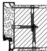
Sarok- és kiegészítő Beépítés tiplis rögzítőelemmel
