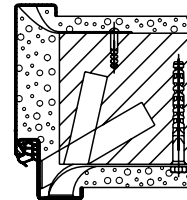
Befoglalótok Beépítés téglafalba Horgony
