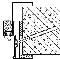
Átlós rögzítés Vario B53 kiegészítővel 2-részes befoglalótként (Gázbeton)
