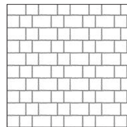
FLORENZ 5 kötés Kőigény (ca): 1 1/2 KŐ 15,63 db/m 2 NORMÁLKŐ 15,63 db/m 2
