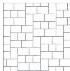
FORTUNA 10 Kőigény (ca): 1 1/2 KŐ 18,6 db/m 2 NORMÁLKŐ 11,2 db/m 2
