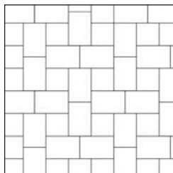
MILANO 3 Keresztkötés Kőigény (ca): TÉGLAKŐ 12,5 db/m 2 NÉGYZETKŐ 6,3 db/m 2
