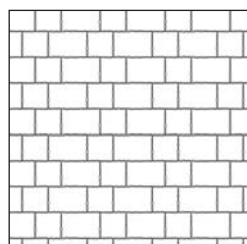
FORTUNA 6 Gótikus kötés Kőigény (ca): 1 1/2 KŐ 15,63 db/m 2 NORMÁLKŐ 15,63 db/m 2
