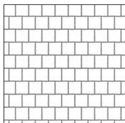
FORTUNA 1 Futókötés Kőigény (ca): NORMÁLKŐ 39,06 db/m 2
