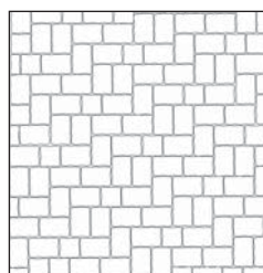
ROMA 5 Kőigény (ca): 1 1/2 KŐ 42,3 db/m 2 NORMÁLKŐ 6,1 db/m 2
