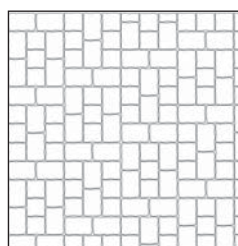
ROMA 10 Kőigény (ca): 1 1/2 KŐ 28,9 db/m 2 NORMÁLKŐ 26,1 db/m 2
