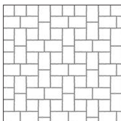
ROMA 1 Keresztkötés Kőigény (ca): 1 1/2 KŐ 34,8 db/m 2 1 1/2 KŐ 17,4 db/m 2
