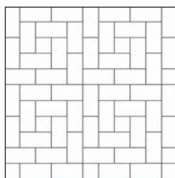
CLASSIC 2 Középkökötés Kőigény (ca): NORMÁLKÓ 48 db/m 2 1/2 KŐ 4 db/m 2
