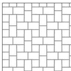
FORTUNA 7 Keresztkötés Kőigény (ca): 1 1/2 KŐ 19,6 db/m 2 NORMÁLKŐ 9,8 db/m 2
