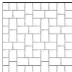
FLORENZ 2 Keresztkötés Kőigény (ca): 1 1/2 KŐ 19,6 db/m 2 NORMÁLKŐ 9,8 db/m 2
