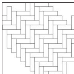
VIA APPIA 2 Halszákkakötés Kőigény (ca): NORMÁLKŐ 68,03 db/m 2
