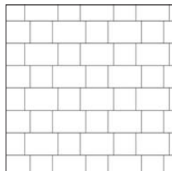
MILANO 4 Gótikus kötés Kőigény (ca): TÉGLAKŐ 10 db/m 2 NÉGYZETKŐ 10 db/m 2
