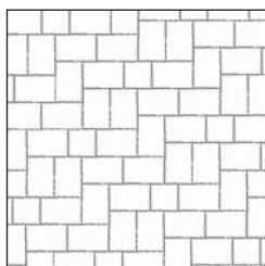
FORTUNA 4 Kőigény (ca): 1 1/2 KŐ 23,8 db/m 2 NORMÁLKŐ 3,4 db/m 2
