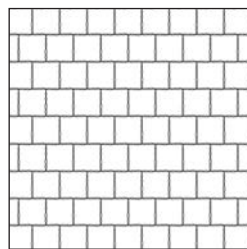
FLORENZ 3 Futókötés Kőigény (ca): NORMÁLKŐ 39,06 db/m 2
