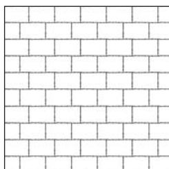
FORTUNA 2 Futókötés Kőigény (ca): 1 1/2 KŐ 26,04 db/m 2
