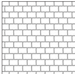
RHODOS 2 Futókötés Kőigény (ca): 1 1/2 KŐ 46,3 db/m 2
