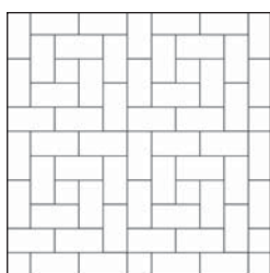
LA TERRAZZA 1 Középkökötés Kőigény (ca): NORMÁLKÓ 48 db/m 2 1/2 KŐ 4 db/m 2
