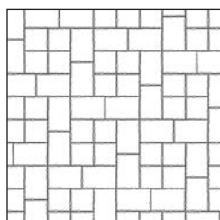
FORTUNA 9 Középkőkötés Kőigény (ca): 1 1/2 KŐ 15,63 db/m 2 NORMÁLKŐ 15,63 db/m 2
