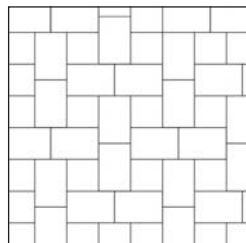
LA PIAZZA 3 Keresztkötés Kőigény (ca): TÉGLAKŐ 12,5 db/m 2 NÉGYZETKŐ 6,3 db/m 2
