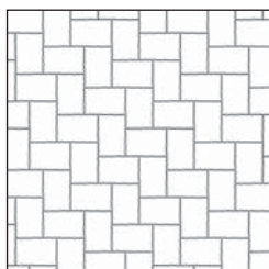
FORTUNA 3 Halszállkakötés Kőigény (ca): 1 1/2 KŐ 26,04 db/m 2
