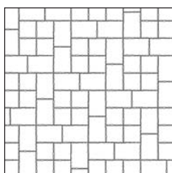
ROMA 7 Középkökötés Kőigény (ca): 1 1/2 KŐ 27,8 db/m 2 NORMÁLKŐ 27,8 db/m 2
