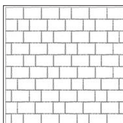
ROMA 6 Bahnverlegung Kőigény (ca): 1 1/2 KŐ 37,9 db/m 2 NORMÁLKŐ 12,6 db/m 2
