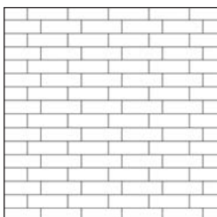
VIA APPIA 1 Futókötés Kőigény (ca): NORMÁLKŐ 68,03 db/m 2
