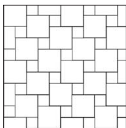
CLASSIC 1 Kőigény (ca): NÉGYZETKŐ 20 db/m 2 1/2 KŐ 20 db/m 2
