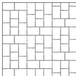
SUAVE 4 Váltókötés Kőigény (ca): 1 1/2 KŐ 19,6 db/m 2 NORMÁLKŐ 9,8 db/m 2
