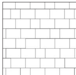
MILANO 2 Futókötés Kőigény (ca): TÉGLAKŐ 13,7 db/m 2 NÉGYZETKŐ 4,5 db/m 2
