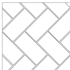
BETONTÉGLA 2 Halszállakakötés Kőigény (ca): NORMALKŐ 32 db/m 2
