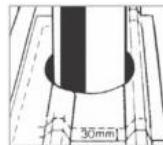
3. Rajzolja fel a Dektite vízzáró gumiharang kontúrját a tetőn. Távolf-tsa el a gumiharangot és jelöljön fel 30 mm-es ráartást.
