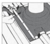
7. Az átlapolandó részek tömítéséhez használja a mellékelt acélzalagokat. Ahol szükséges, vágja le a felesleges széleket.
