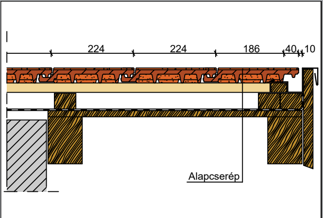
Oromszegély, alapcseréppel
