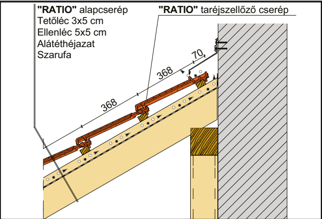
Falcsatlakozás
