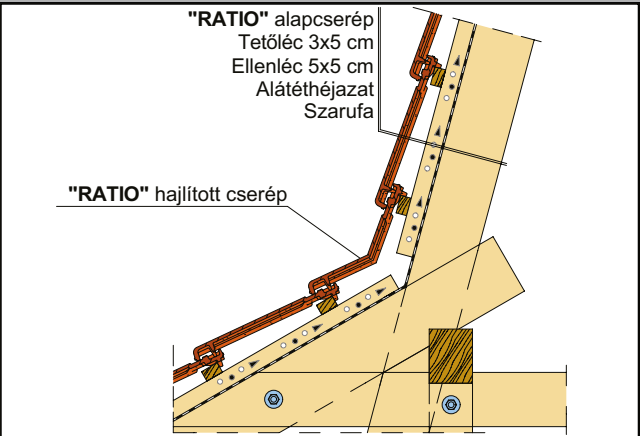
Hajlítót cserép
