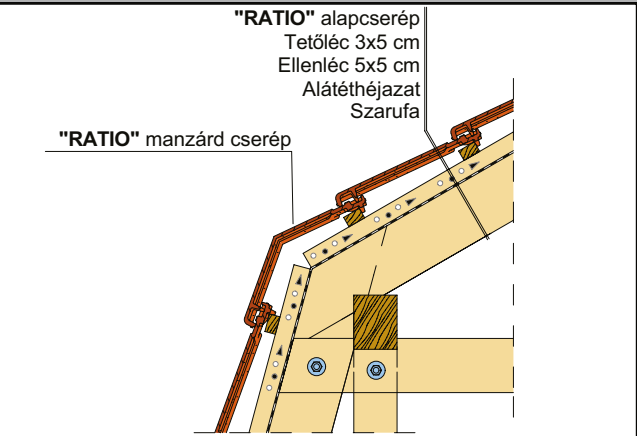
Manzárd cserép
