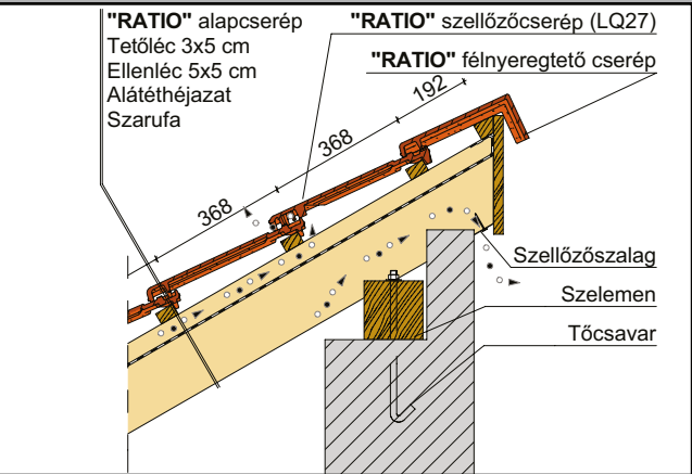
Félnyeregterítő
