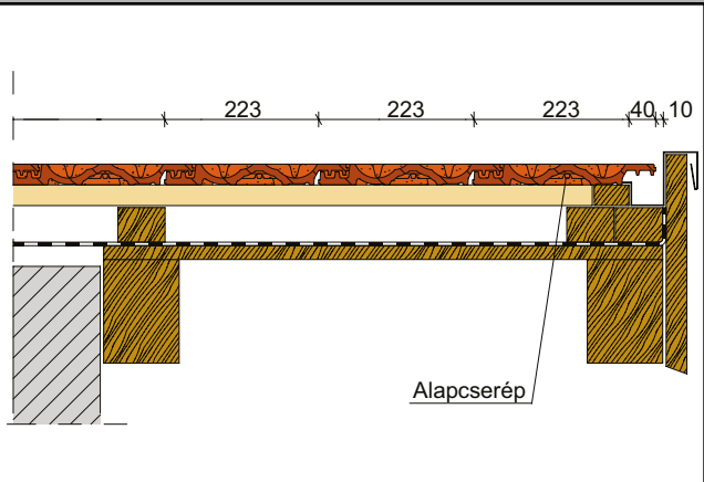
Oromszegély, alapcseréppel
