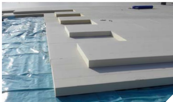
Fokozott hőszigetelés, PIR táblák két rétegben fektetve
